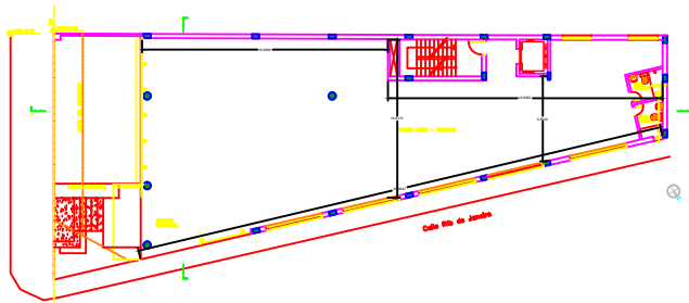
PLANTA ARQUITECTÓNICA – NIVEL +1,12 Escala 1:100
